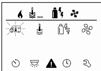
Fig. 101 : Afficheur du niveau de réglage
