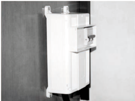
Fig. 3 : Interrupteur principal (disjoncteur différentiel)
