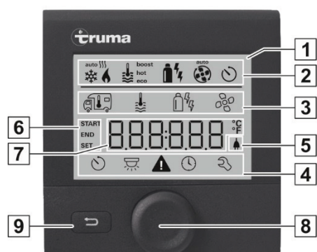
Fig. 98: Unité de commande digitale TRUMA CP Plus
